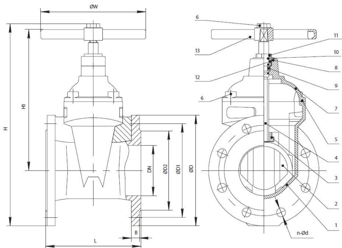
Рисунок 1. Задвижки DN 50-300
