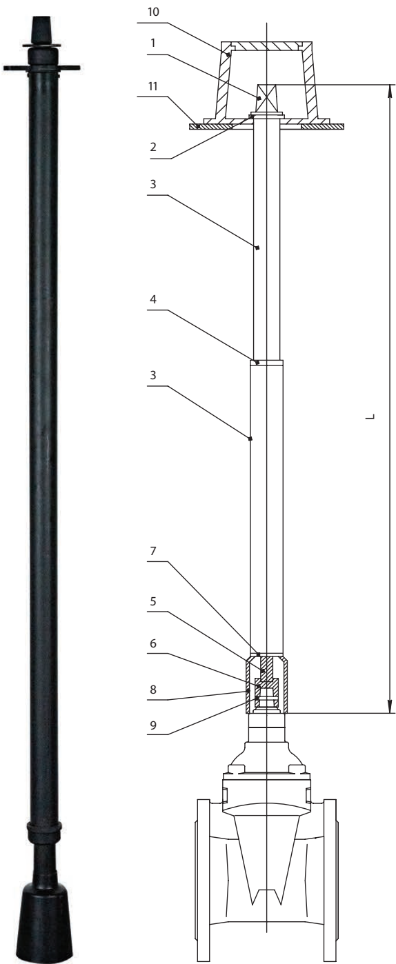
Комплект для бесколодезной установки запорной арматуры
