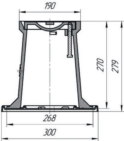
Ковер и опорная плита часть комплекта бесколодезной установки
