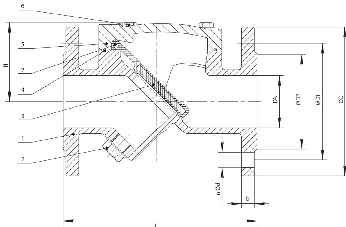
Рисунок 1. Конструкция клапана
