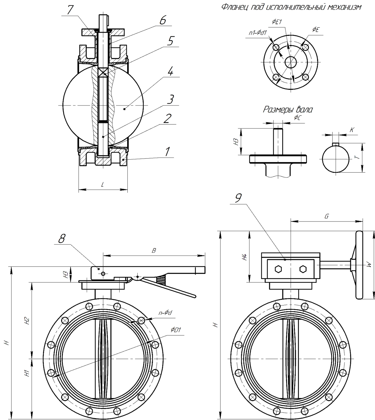
Рисунок 1. Затвор 021F.Y с рукояткой DN50-300 и редуктором DN50-300
