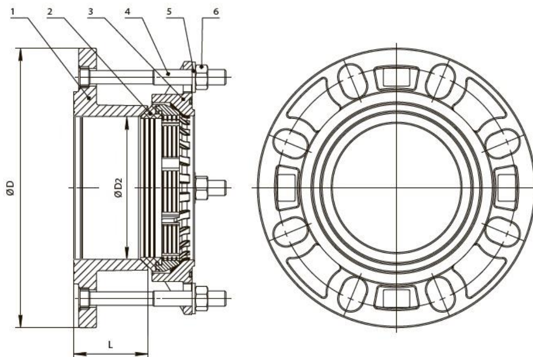
Рисунок 1. Фланец обжимной фиксирующий DN50-300(315)
