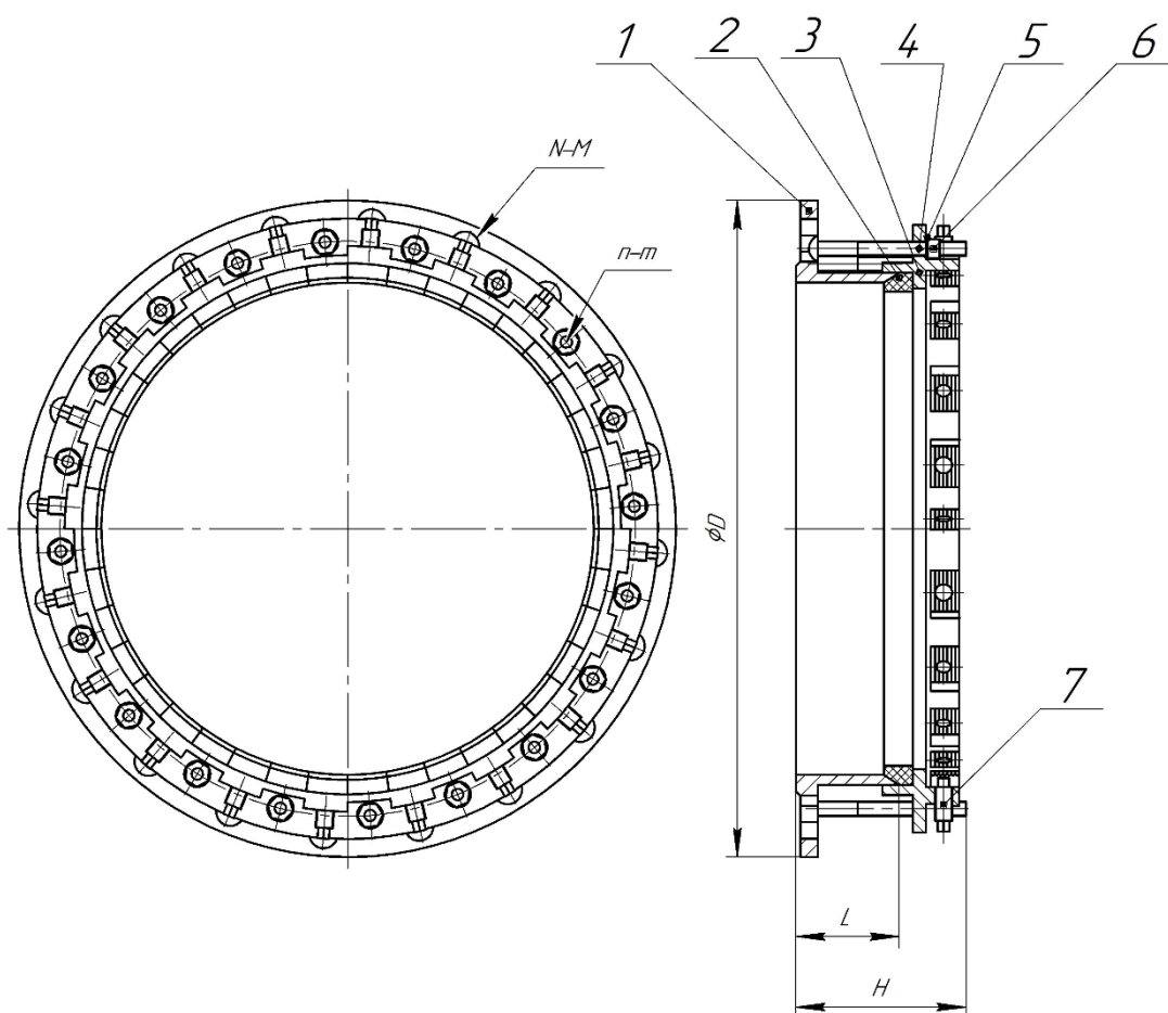
Рисунок 2. Фланец обжимной фиксирующий DN300(355)-1200
